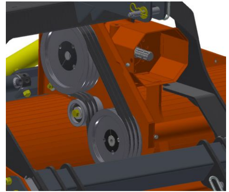
Zusätzliche Riemenscheibe für verbesserten Halt und weniger Verschleiß der mittleren Keilriemen
