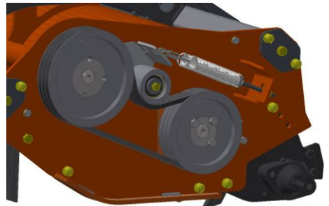
Automatisches Spannen der Rotorantriebskeilriemen
